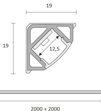
LIMENTE LED-CORNER
