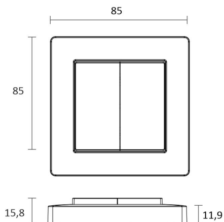
LIMENTE SMART 522
