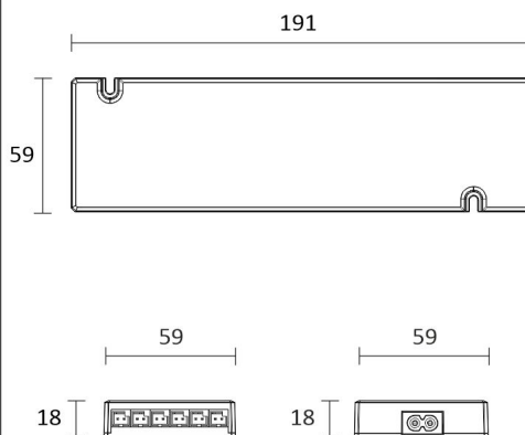
LIMENTE 28060
